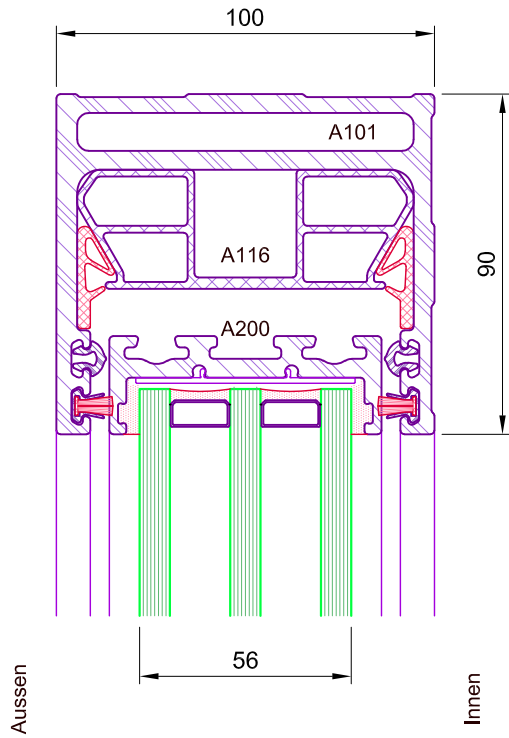
Schnitt durch Schiebeflügel
