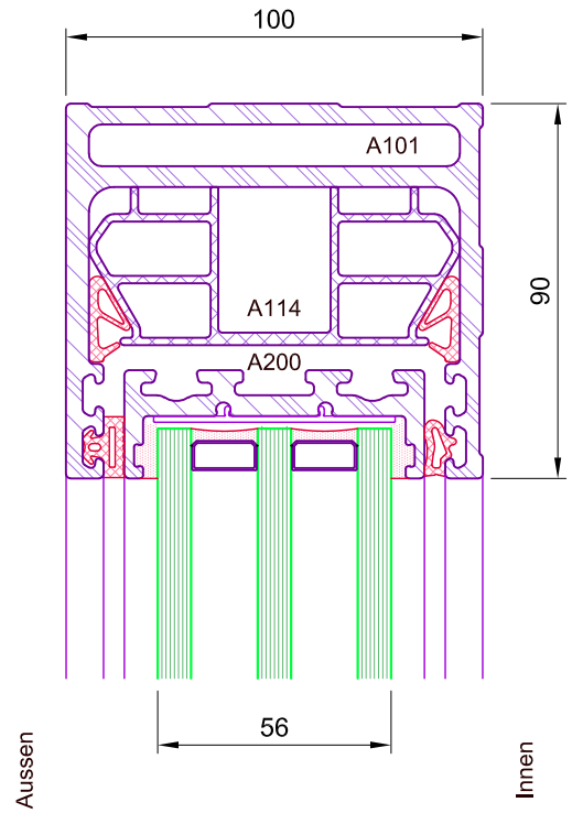
Schnitt durch Festelement
