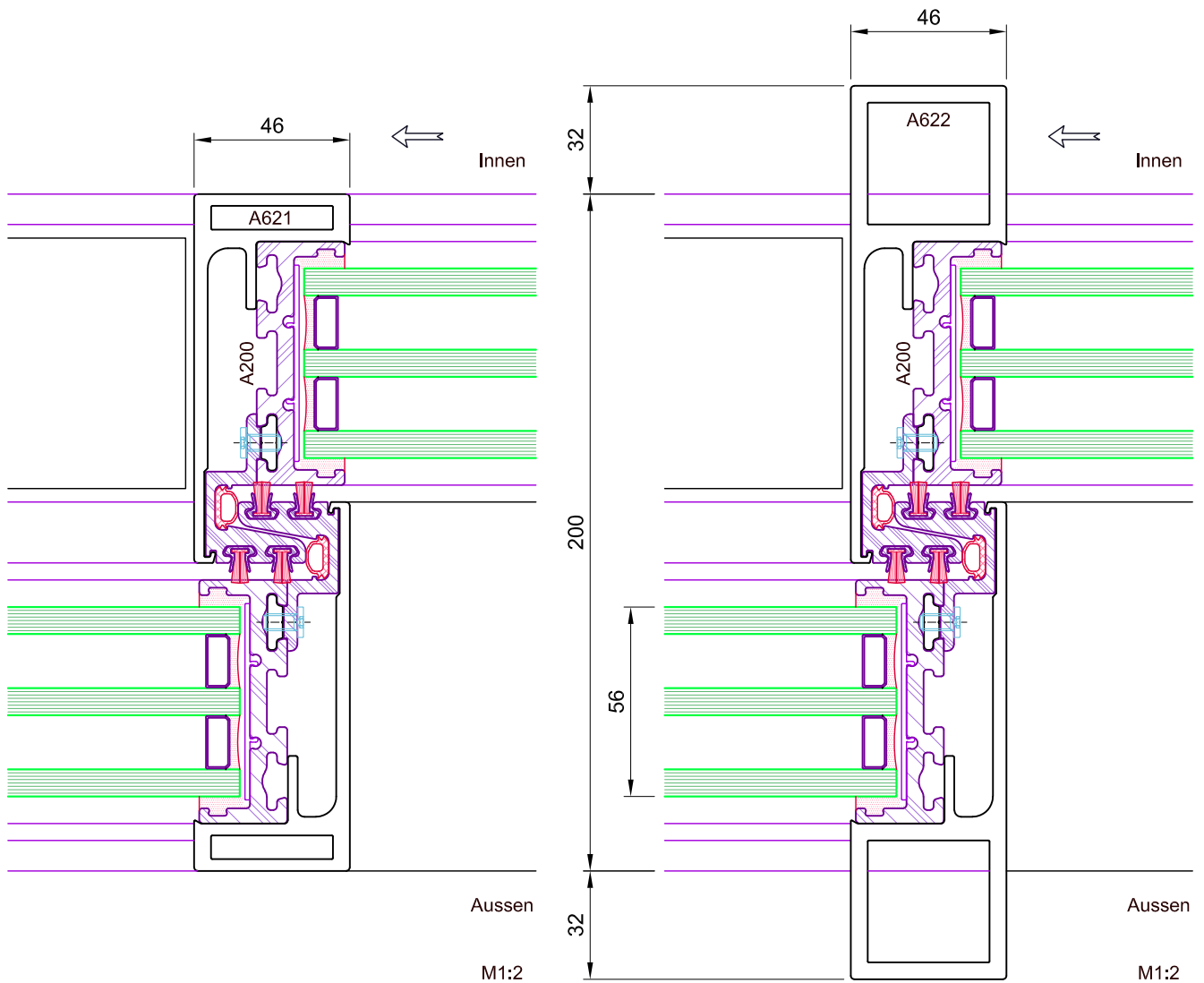
Mittelprofil U-förmig Grösse S 46mm
